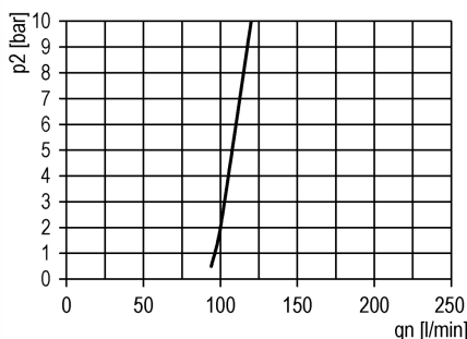
Öleransprechgrenze
